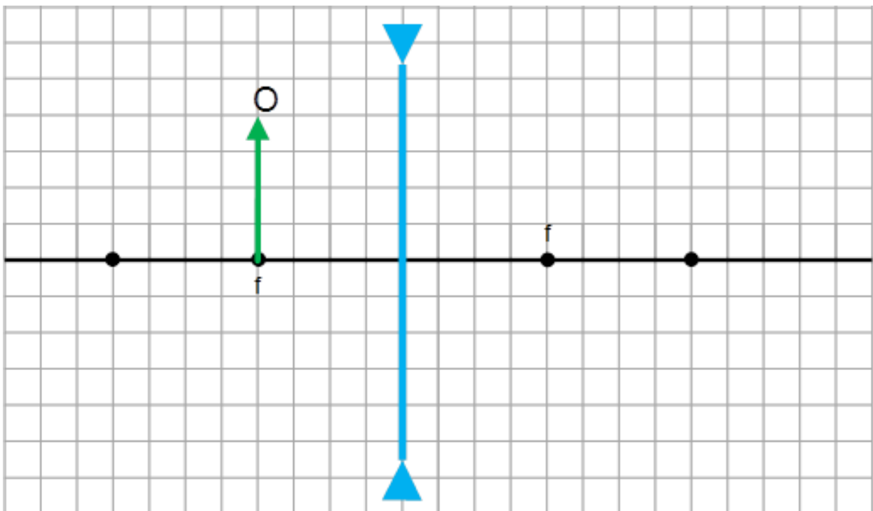
Figura 8: Objeto no foco
