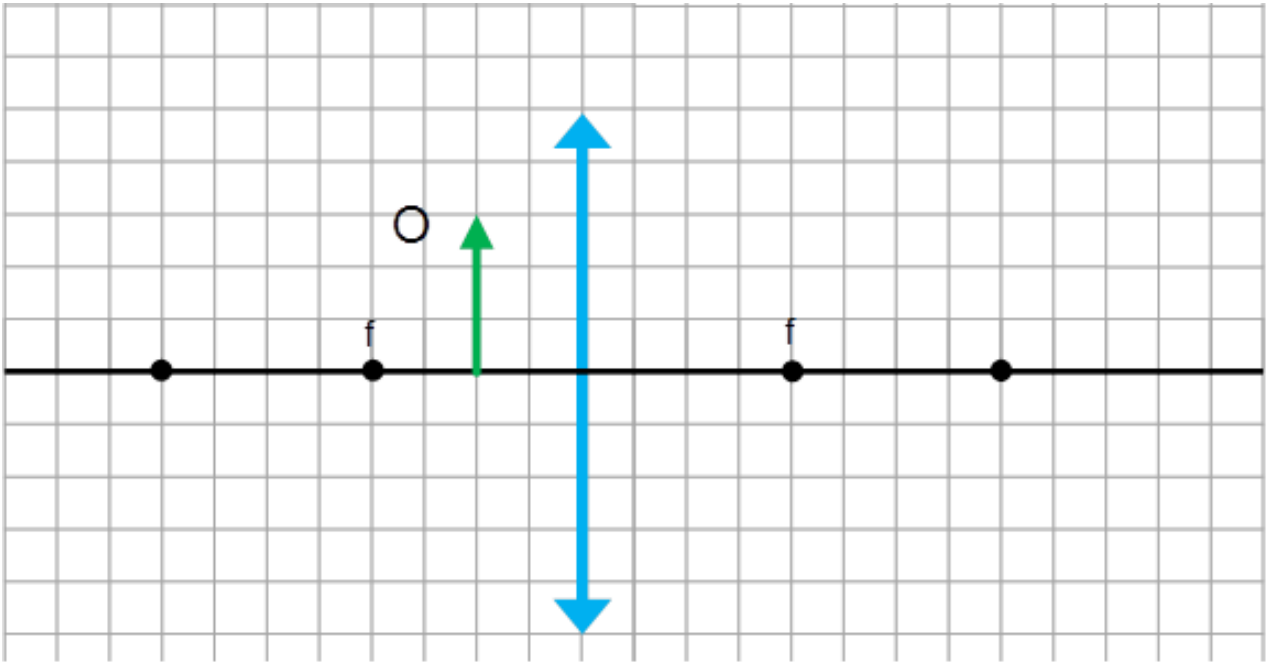
Figura 1: Objeto entre o vértice e o foco
